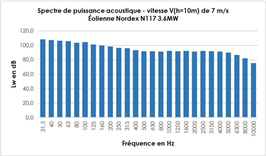
Figure 8. Graphe des niveaux de puissance acoustique d'une Nordex N117-3.6MW par bande de tiers d'octave à la vitesse de 7 m/s (à la hauteur standardisée de 10 m)
