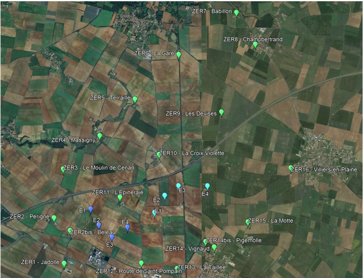
Figure 9. Implantation des projets de renouvellement de la ferme éolienne de Benet et de La Croix Violette
