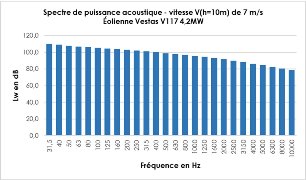
Figure 6. Graphe des niveaux de puissance acoustique d'une Vestas V117-4.2MW par bande de tiers d'octave à la vitesse de 7 m/s (à la hauteur standardisée de 10 m)
