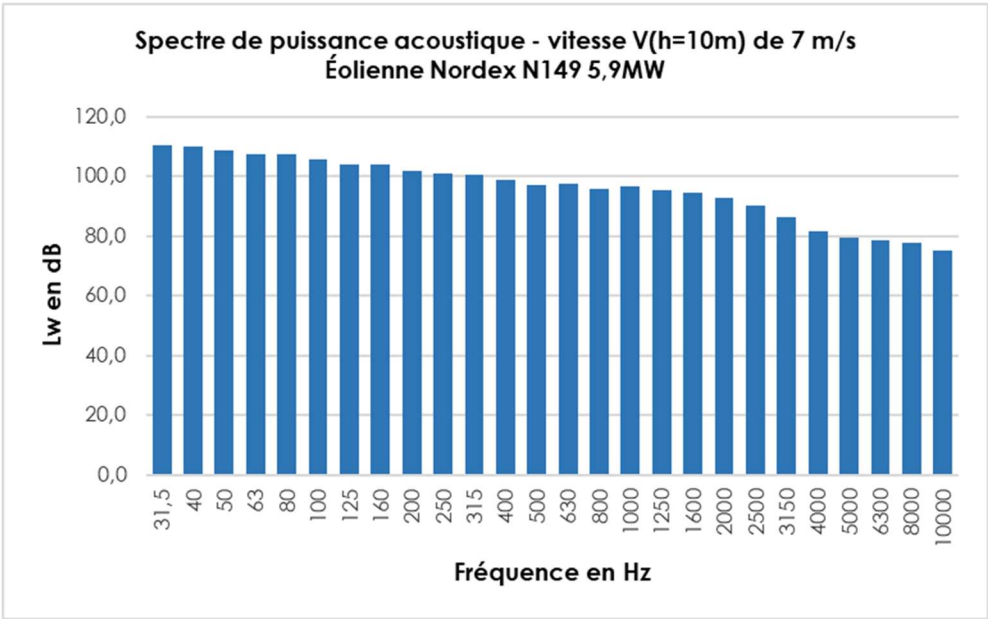
Figure 7. Graphe des niveaux de puissance acoustique d'une Nordex N149-5.9MW par bande de tiers d'octave à la vitesse de 7 m/s (à la hauteur standardisée de 10 m)
