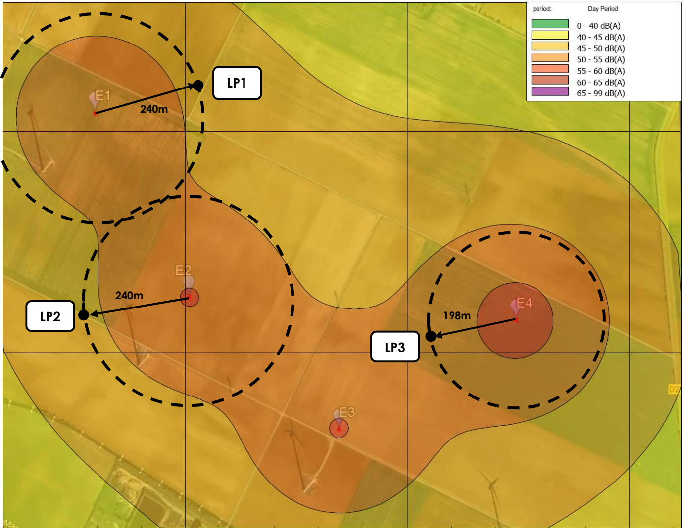
Figure 4. Cartographie sonore – Projet de renouvellement de la ferme éolienne de Benet
