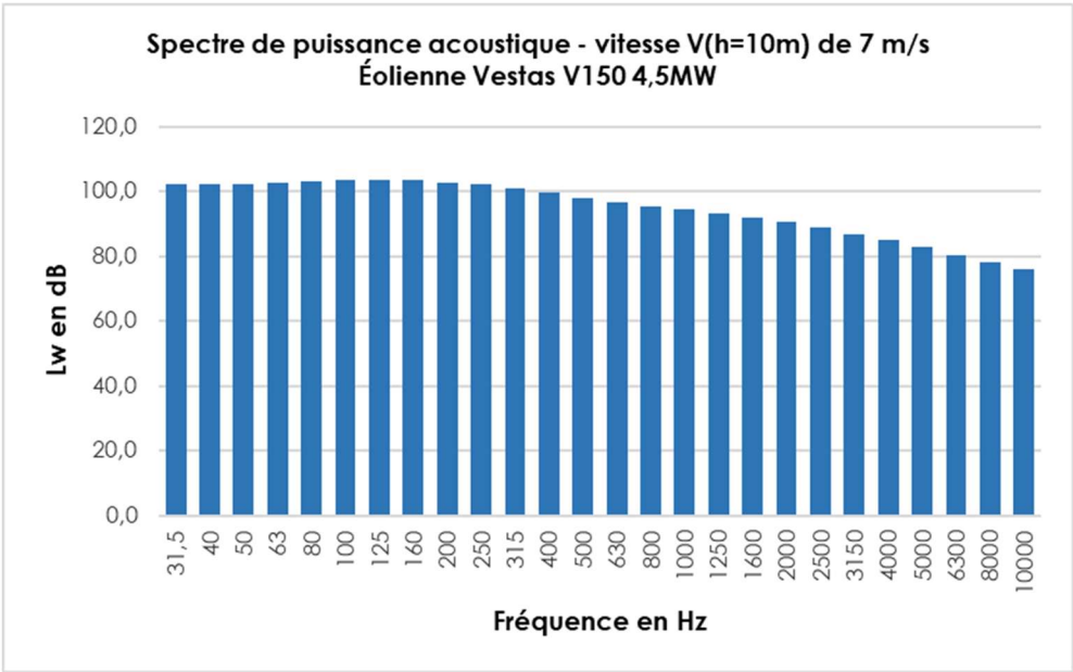
Figure 5. Graphe des niveaux de puissance acoustique d'une Vestas V150-4.5MW par bande de tiers d'octave à la vitesse de 7 m/s (à la hauteur standardisée de 10 m)
